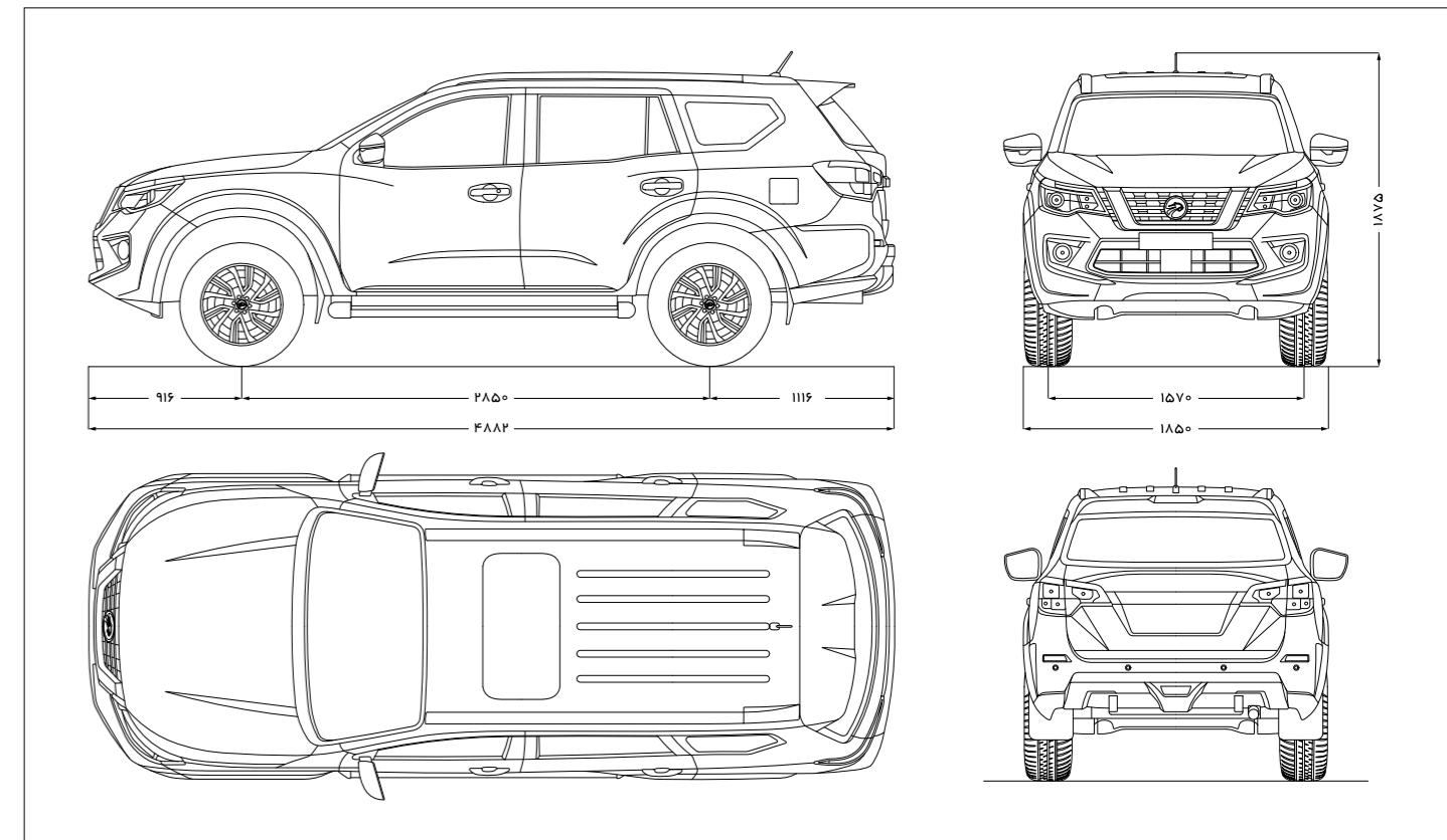
ابعاد کلی خودرو ( میلی متر )
